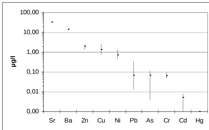
Figur 30. Konsentrasjoner av metaller i Mjøsa. Figuren viser middelværddier og variasjonsbredder for samtlige prøver og dyp i 2006. Ved konsentrasjoner lavere enn deteksjonsgrensene har vi brukt 0,5 ganger deteksjonsgrensene for framstilling av figuren.
