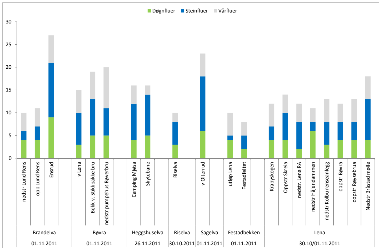
Figur 13. Biologisk mangfold uttrykt ved antall taksa av døgnfluer, steinfluer og vårfluer (EPT)
