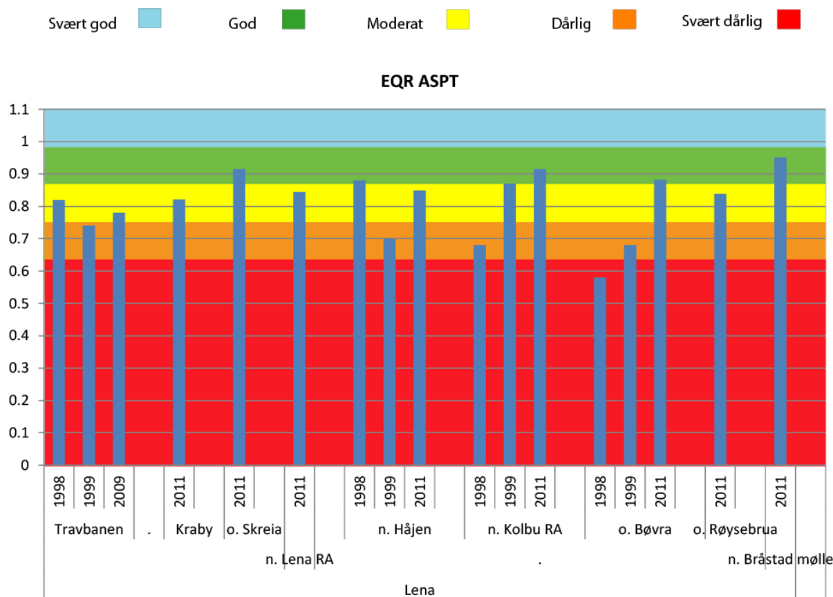
Figur 9. Økologisk tilstand i ulike deler av Lena høsten 2011 samt 1998 og 1999 for enkelte stasjoner.
