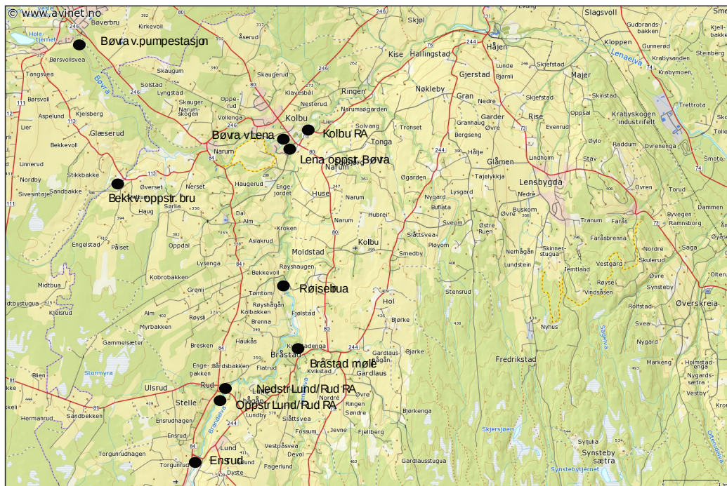
Figur 2. Bunndyrstasjoner fra øvre del av Lenavassdraget inkludert Bøvre.
