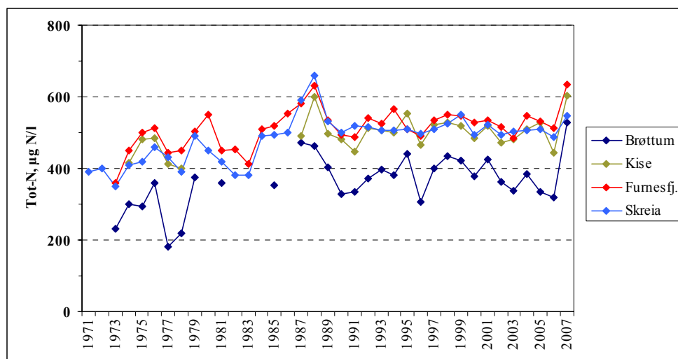
Figur 11. Tidsutviklingen i middelverdier av total-nitrogen (vertikalserier fra overflata til bunnen) fra observasjoner på sen vinteren i perioden 1971-2007.
