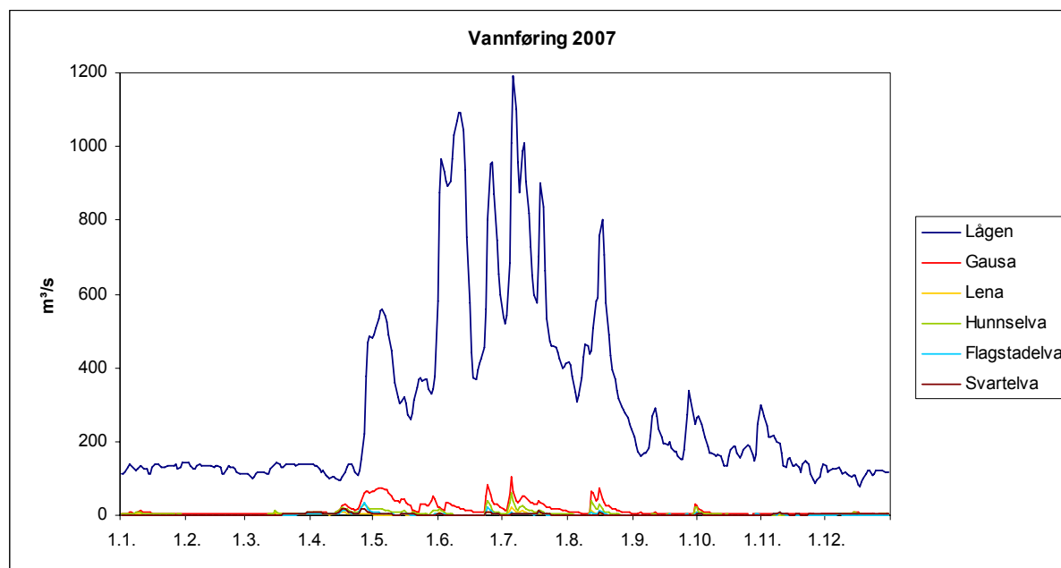
Figur 34. Vannføring i de 6 viktigste tilløpselvene til Mjøsa i 2007.
