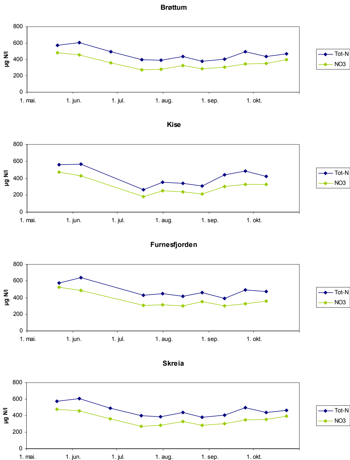
Figur 13. Konsentrasjoner av total-nitrogen og nitrat ved 4 stasjoner i Mjøsa (0-10 m) i 2007.
