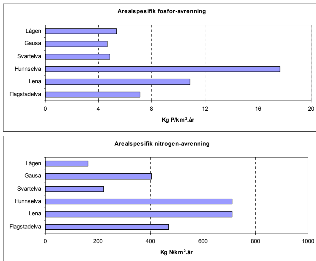
Figur 38. Areal spesif avrenning av fosfor og nitrogen i 2007.
