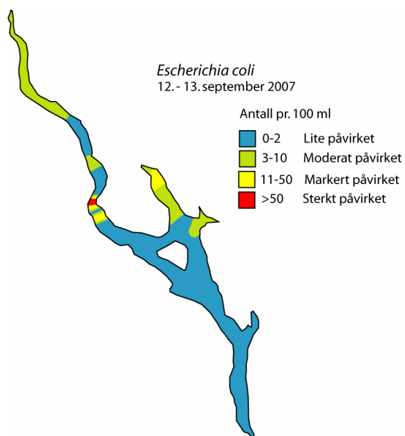
Figur 31. Konsentrasjonen av E. coli i Mjøsas øvre vannlag vurdert på grunnlag av resultatene fra 3 prøvedyp (se figur ovenfor). For nærmere beskrivelse av forholdene, se sammendragkapitlet.
