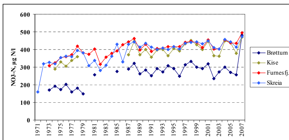
Figur 12. Tidsutviklingen i middelverdier av nitrat (vertikalserier fra overflata til bunnen) fra observasjoner på sen vinteren i perioden 1971-2007.
