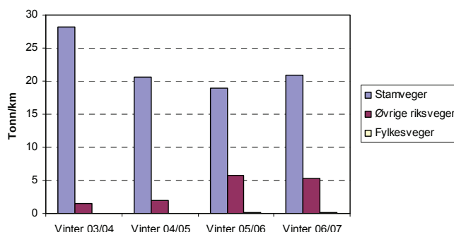
Figur 5. Saltforbruk på veier i Gjøvik og Toten (kontrakt 0501) i perioden fra vinteren 2003/04 til vinteren 2006/07 (Kilde: Winter-Larsen og Melve 2009).
