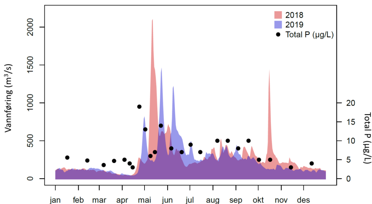
Figur 32. Døgnmiddelvannføring ( \text{m}^3/\text{s} ) og konsentrasjoner av Tot-P i vannprøver fra Lågen gjennom 2019. Til sammenlikning er vannføringen gjennom 2018 vist med lyserød farge.
