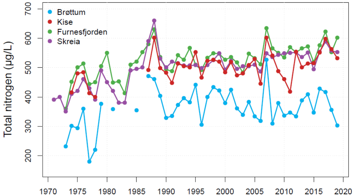
Figur 15. Tidsserier i konsentrasjoner av total nitrogen på senvinteren i perioden 1971-2019 (basert på middelverdier av konsentrasjonen i vannprøver fra vertikalsier fra overflaten til nær bunnen).
