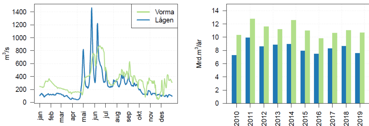
Figur 4. Vannføring i Lågen (vannmerke Losna) og i Vorma ved Minnesund i 2019 (venstre panel). Årlig vanntransport med Lågen og Vorma i perioden 2010-2019 (mrd. = milliarder) (høyre panel). Basert på data fra NVE og Eidsiva kraft.
