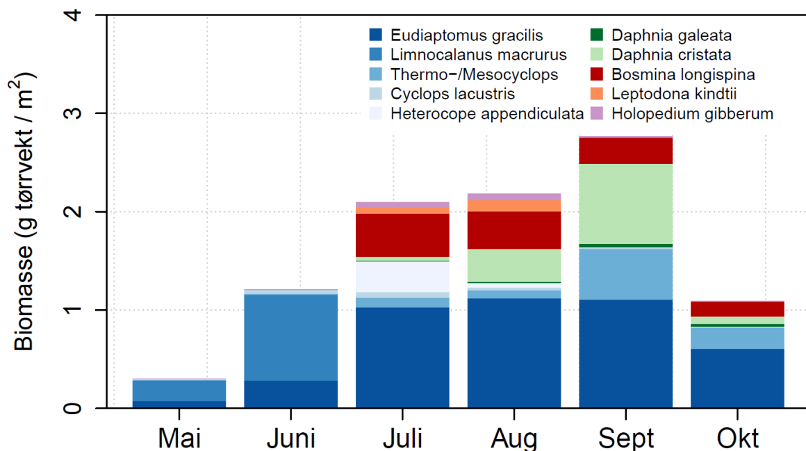
Figur 27. Sesongutviklingen i biomasser av de viktigste artene innen krepsdyrplanktonet ved stasjon Skreia i 2019 basert på kvantitativ prøvetaking med Schindler-felle. Biomasser er gitt som g tørrvekt pr. m 2 for sjiktet 0-50 m.
