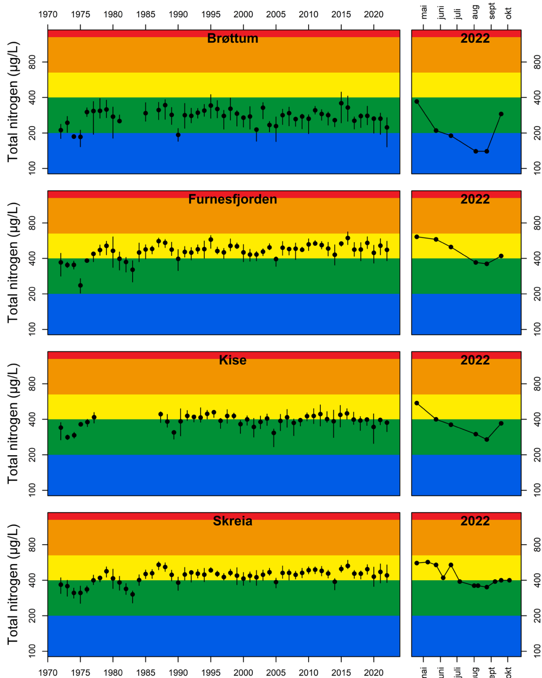
Figur 9. Tidsutviklingen i middelverdier for Tot-N i mai-oktober i sjiktet 0–10 m i perioden 1972–2022. Se Figur 7 for utfyllende figurtekst.
