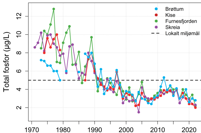
Figur 6. Tidsutvikling i konsentrasjoner av Tot-P i dypserier på senvinteren/tidlig vår (fra isen eller i tidlig i mai i år uten is). Punktene representerer middelverdier for prøver fra 0–60 m ved Brøttum (blå), 0–200 m ved Kise (rød), 0–60 m i Furnesfjorden (grønn) og 0-ca. 428 m ved Skreia (lilla).
