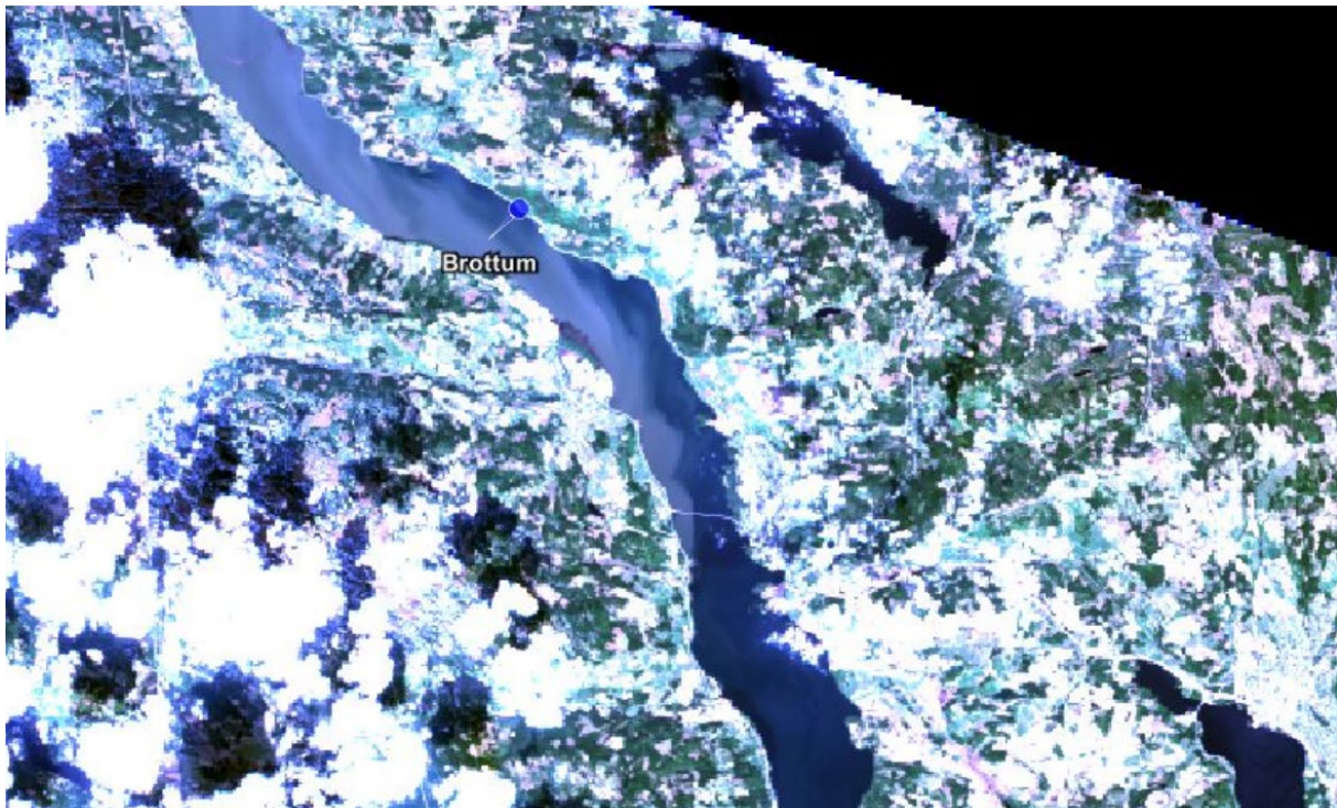
Figur 3. Satellittbilde (RGB) som viser deler av nordre deler av Mjøsa 16 mai 2018, like etter flomtoppen i Lågen. Floppen svært kraftig dette året pga. ekstrem varme på Østlandet. En kan tydelig tungen med partikkelrikt vann (i hovedsak brepartikler) som strekker seg sørover. Bildet er hentet fra satellitten Sentinel 2 den 16 mai 2018 (sakset fra Ledang, Harvey og Marty, 2019).
