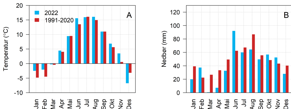
Figur 2. A) Gjennomsnittlig lufttemperatur og B) sum av nedbør (mm) pr. måned ved Kise meteorologiske stasjon i 2022 (blå søyler). Normaler for perioden 1991–2020 er vist med røde søyler. Dataene er innhentet fra NIBIO, Landbruksmeteorologisk tjeneste (LMT).
